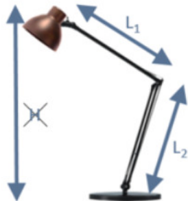
Leuchte (mit Gelenken) Äußere Abmessung: Der größere Wert von L_1 oder L_2 (nicht H)
