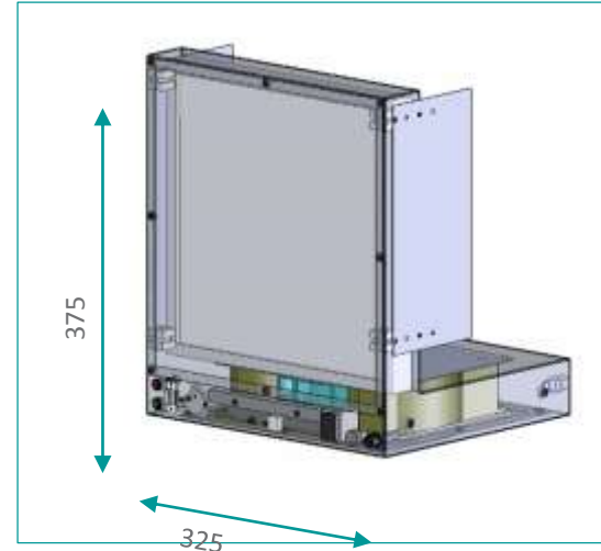
Robot-FFU
